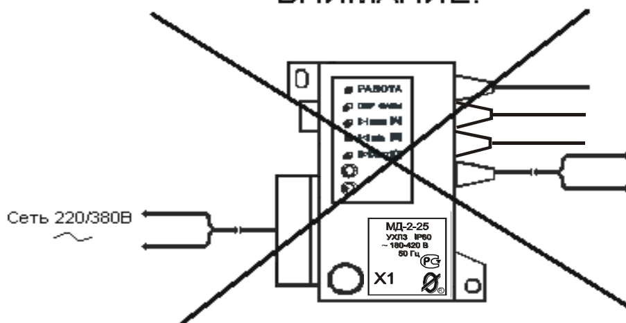
Неправильное подключение - ведет к выходу ключа управления из строя
